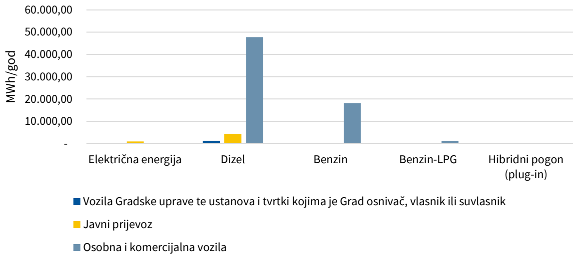
Grafikon 8. Prikaz potrošnje energenata po podsektorima unutar sektora prometa u 2024. godini
