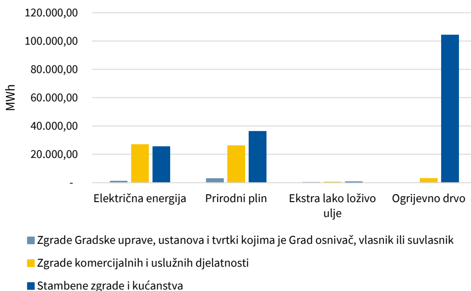
Grafikon 1. Prikaz potrošnje energenata po podsektorima unutar sektora zgradarstva u 2024. godini
