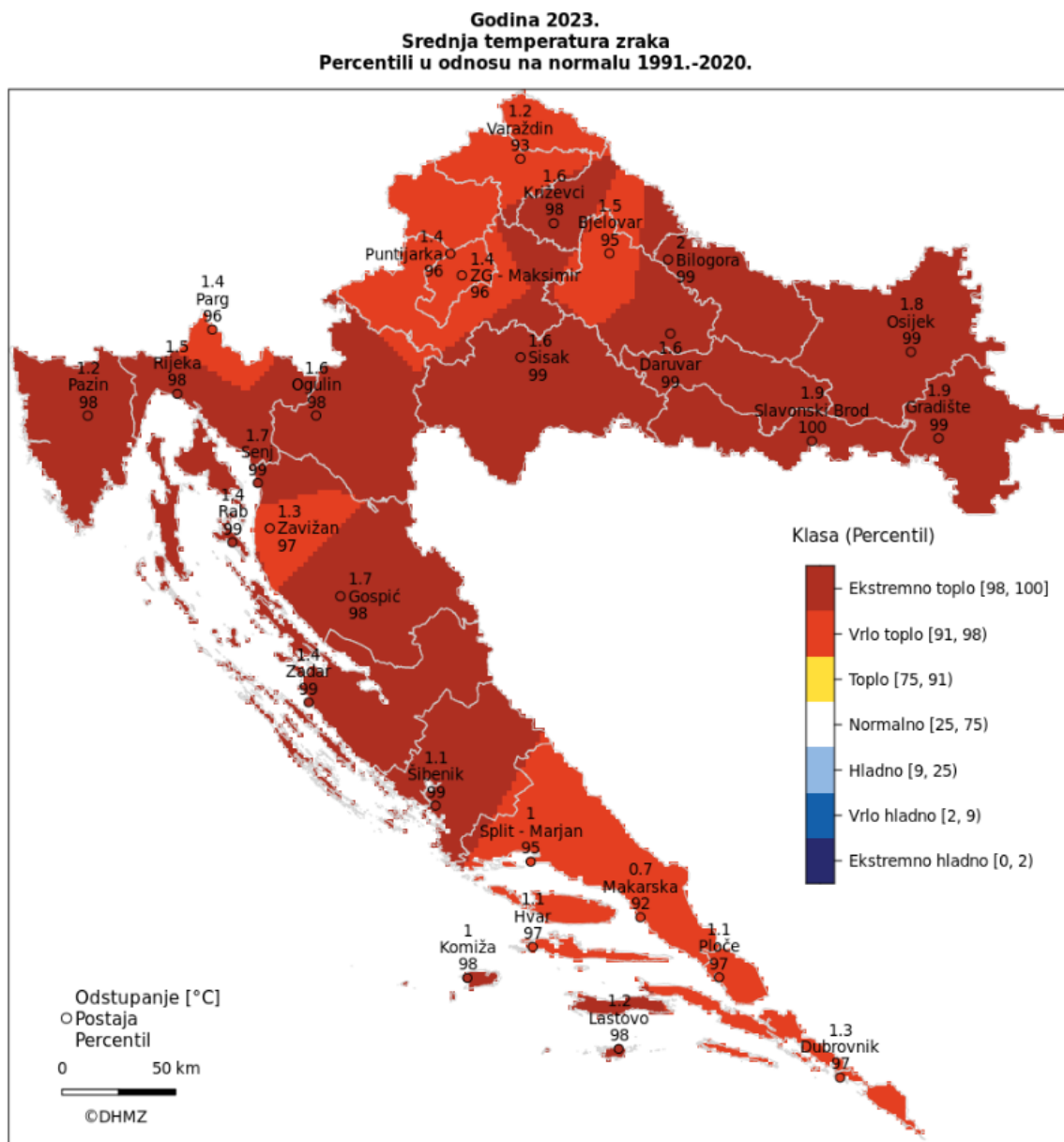
Slika 1: Odstupanje srednje mjesečne temperature zraka (° C) od višegodišnjeg prosjeka za razdoblje 1961.-1990. godine za Hrvatsku za 2023. godinu
