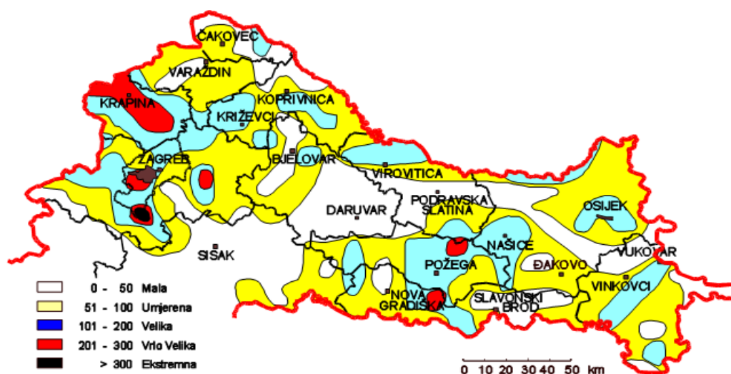
Slika 5: Prostorna raspodjela indeksa ugroženosti od pojave tuče sa štetom na branjenom području Hrvatske. 1981–2000.
