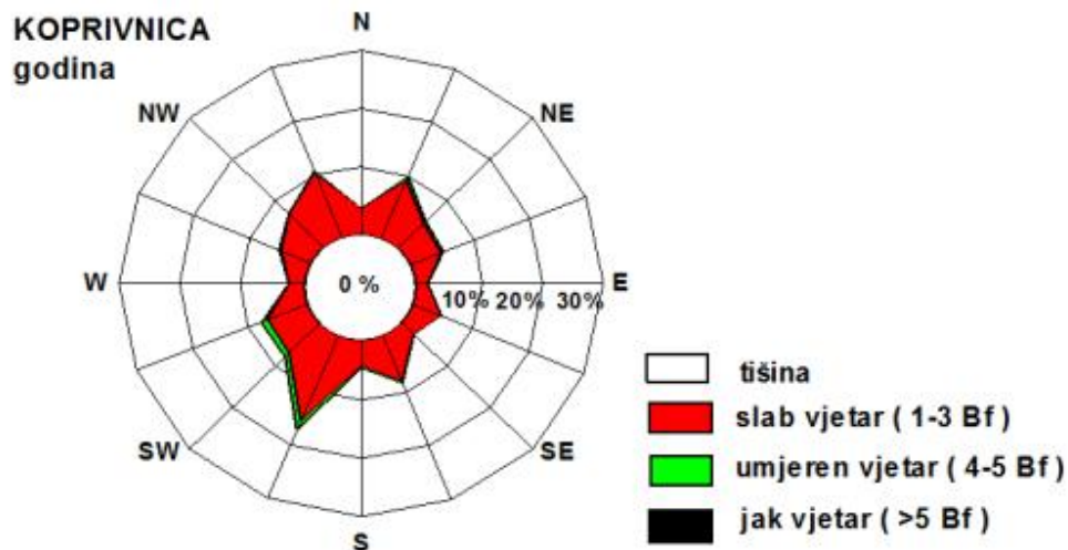
Slika 4: Godišnja ruža vjetrova Koprivničko-križevačke županije Izvor podataka: DHMZ-meteorološke podloge
